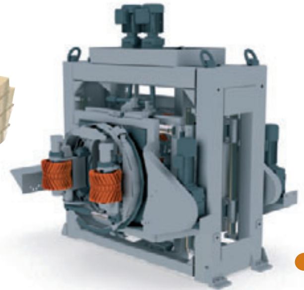
Hög måttnoggrannhet och matningshastighet med HewSaw Log-In
