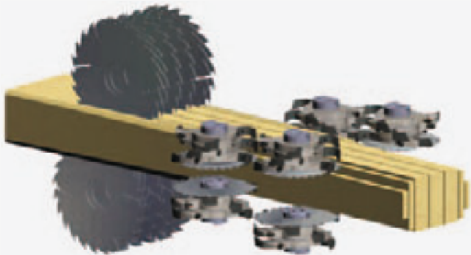
Delningssågen kurvsågar blocket och kantar upp till fyra optimerade kantbrädor.
